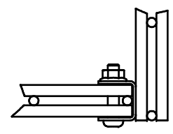
A ( 1 : 2 )
