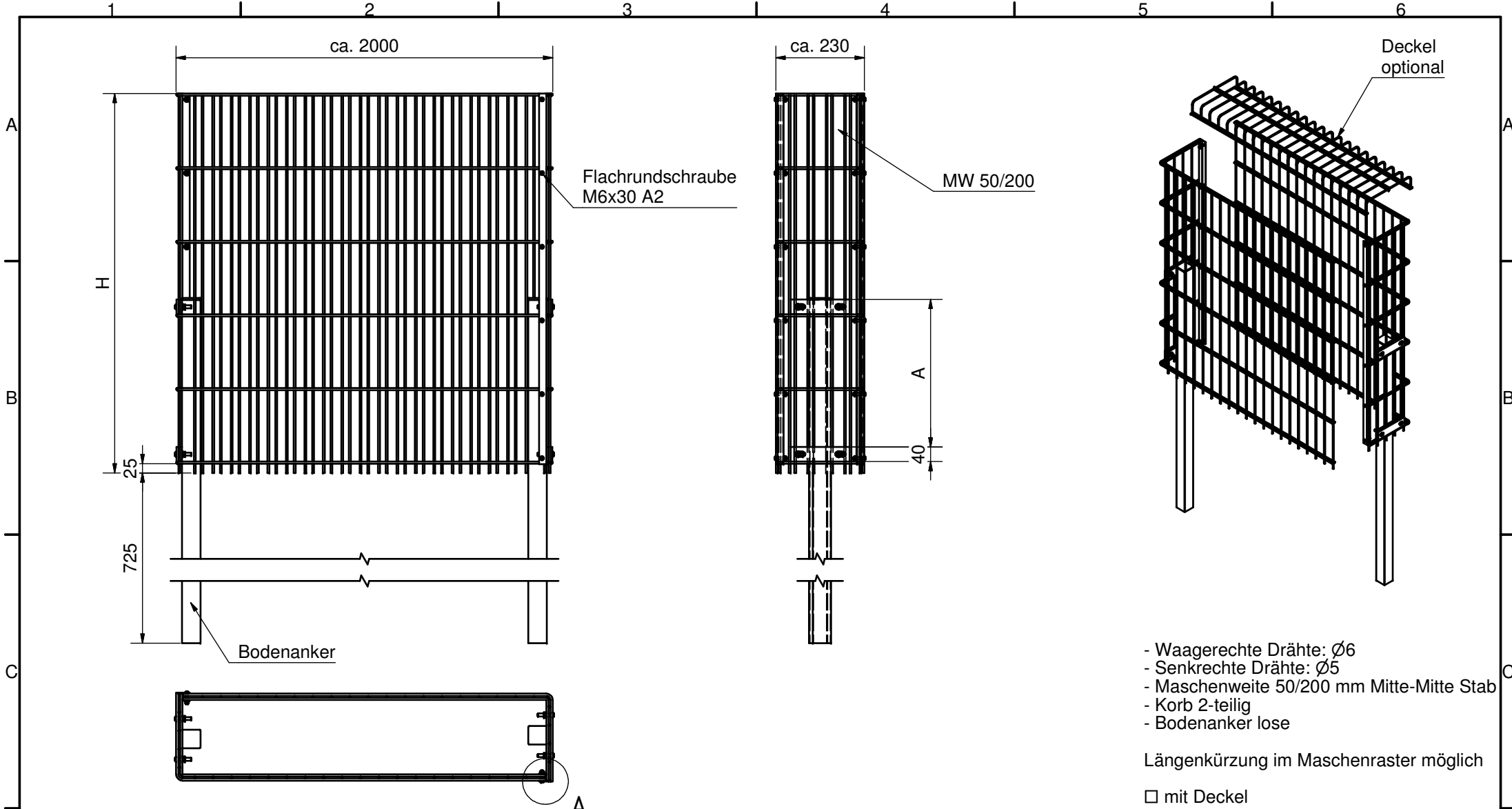
Abmaße Bodenanker
